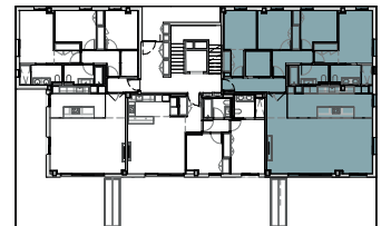
PLANTA BAIXA
